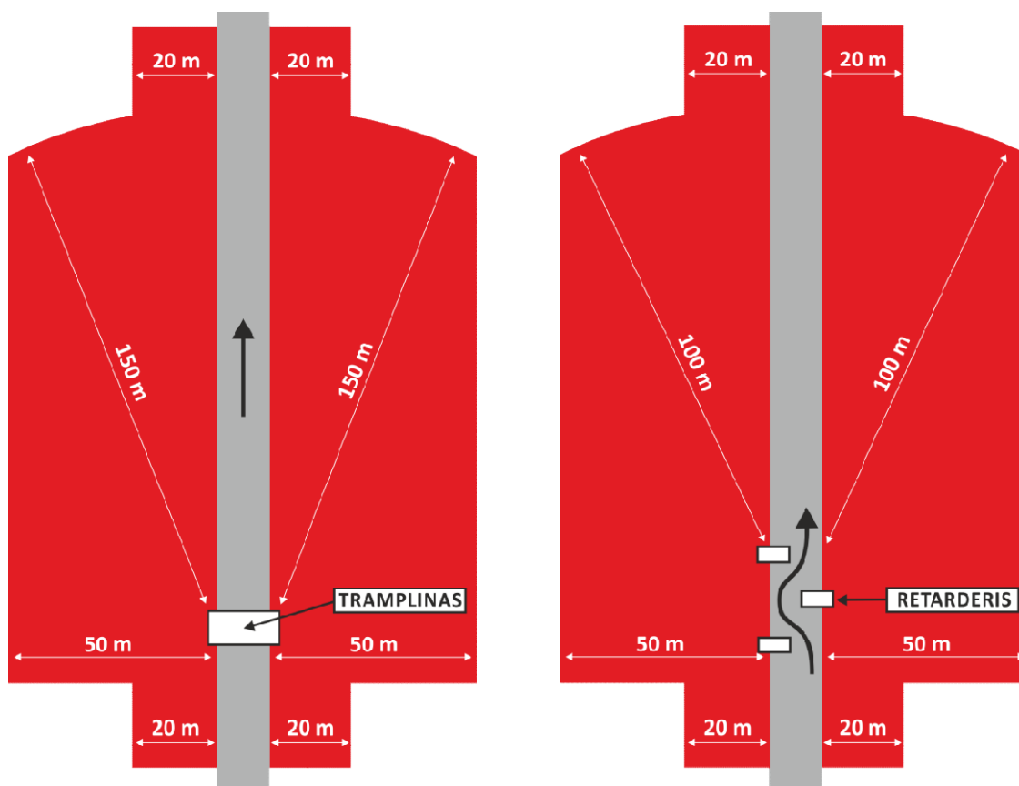
Tramplinas ir retarderis tiesioje trasos atkarpoje
